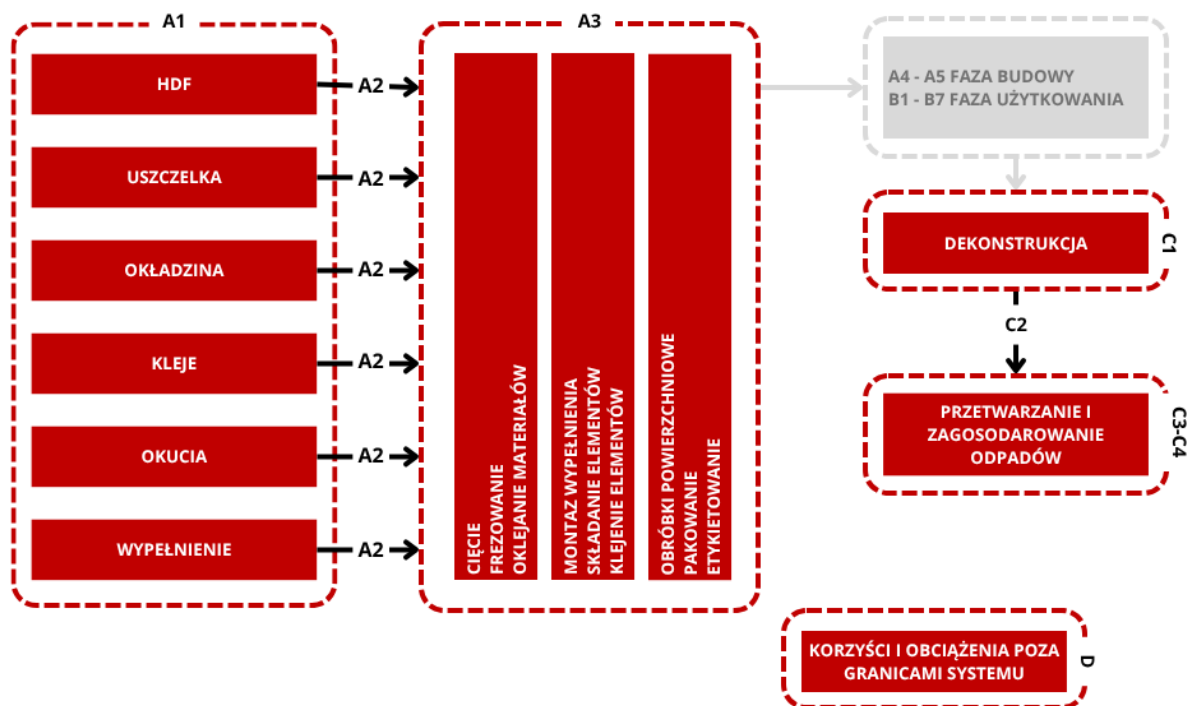
Rysunek 5.1: Granice systemu dla charakterystyki środowiskowej drzwi technicznych
